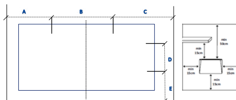
Ophangbeugel achterkant
